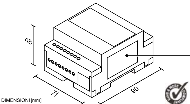
DIMENSIONI [mm]
